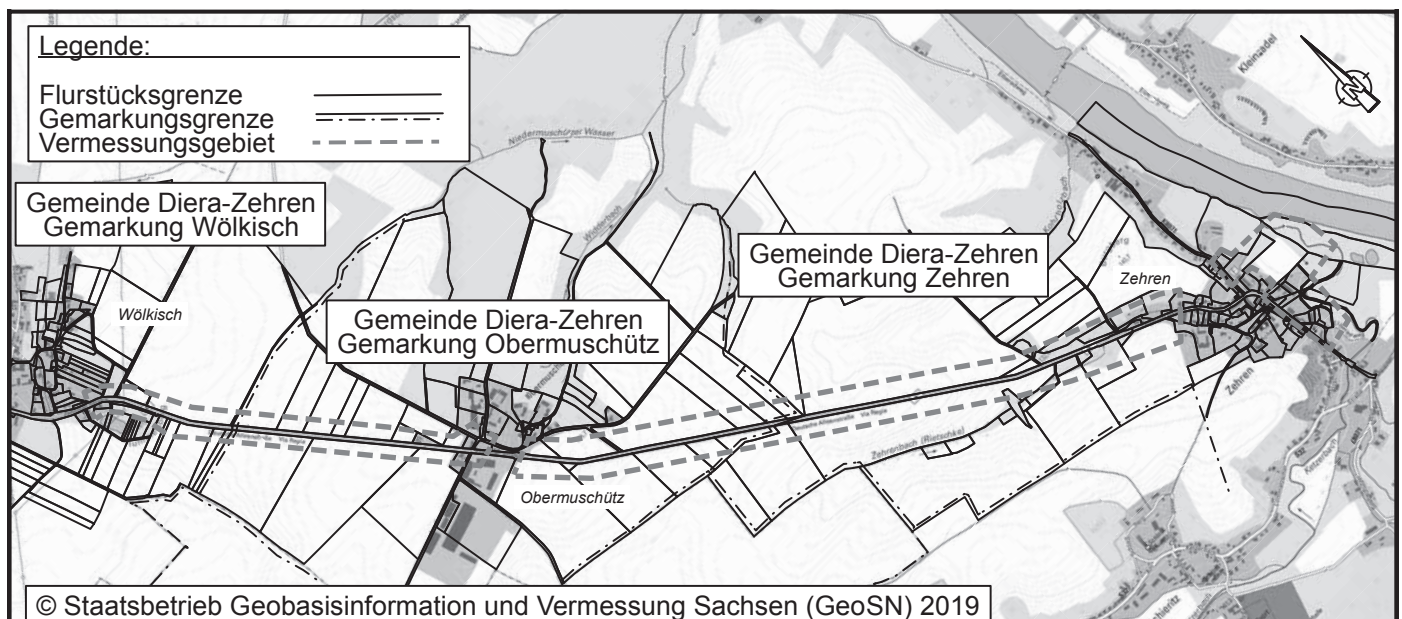
Übersichtslageplan
